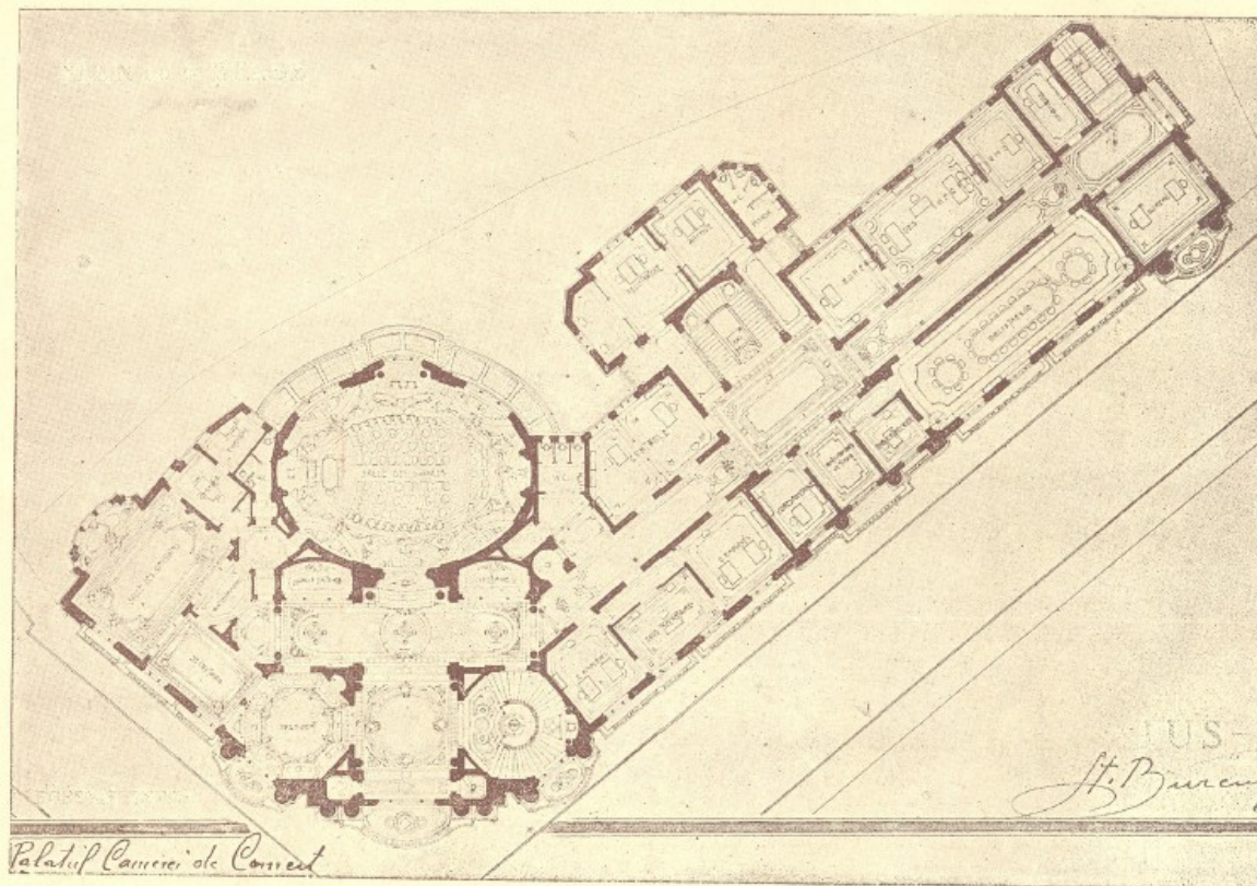
Planul Parterului.
